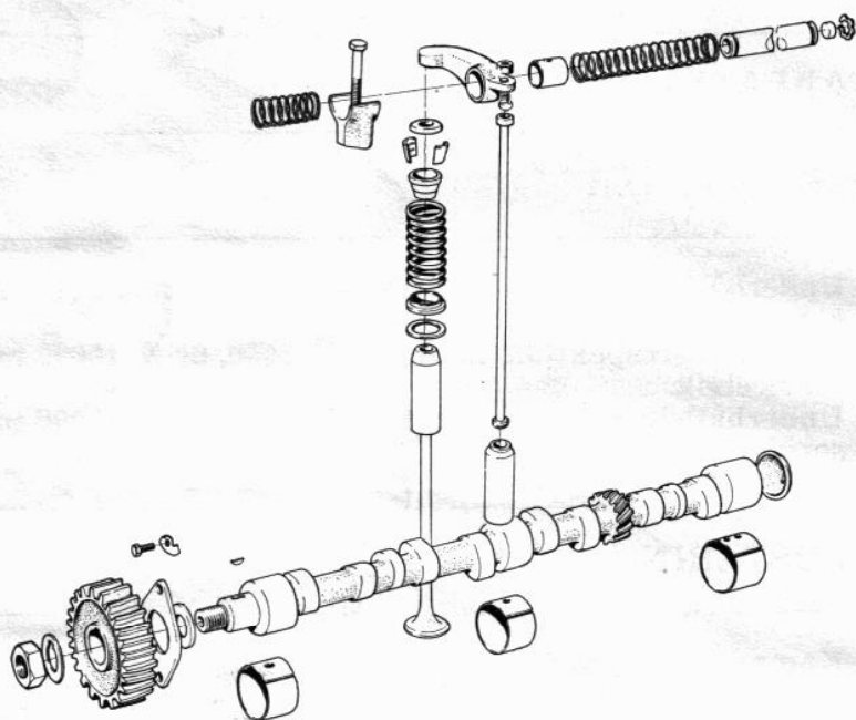
Ventilmekanism
