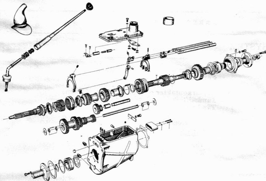
Växellåda, M-4
