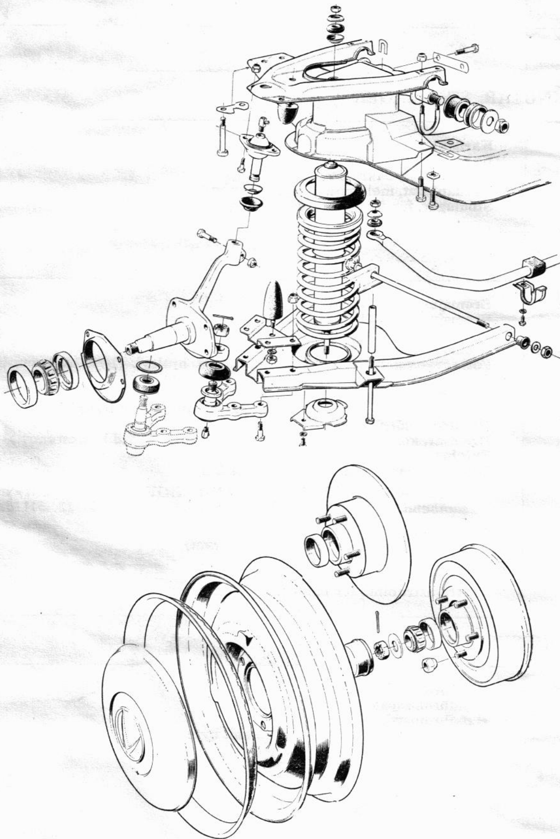
Framvagn
