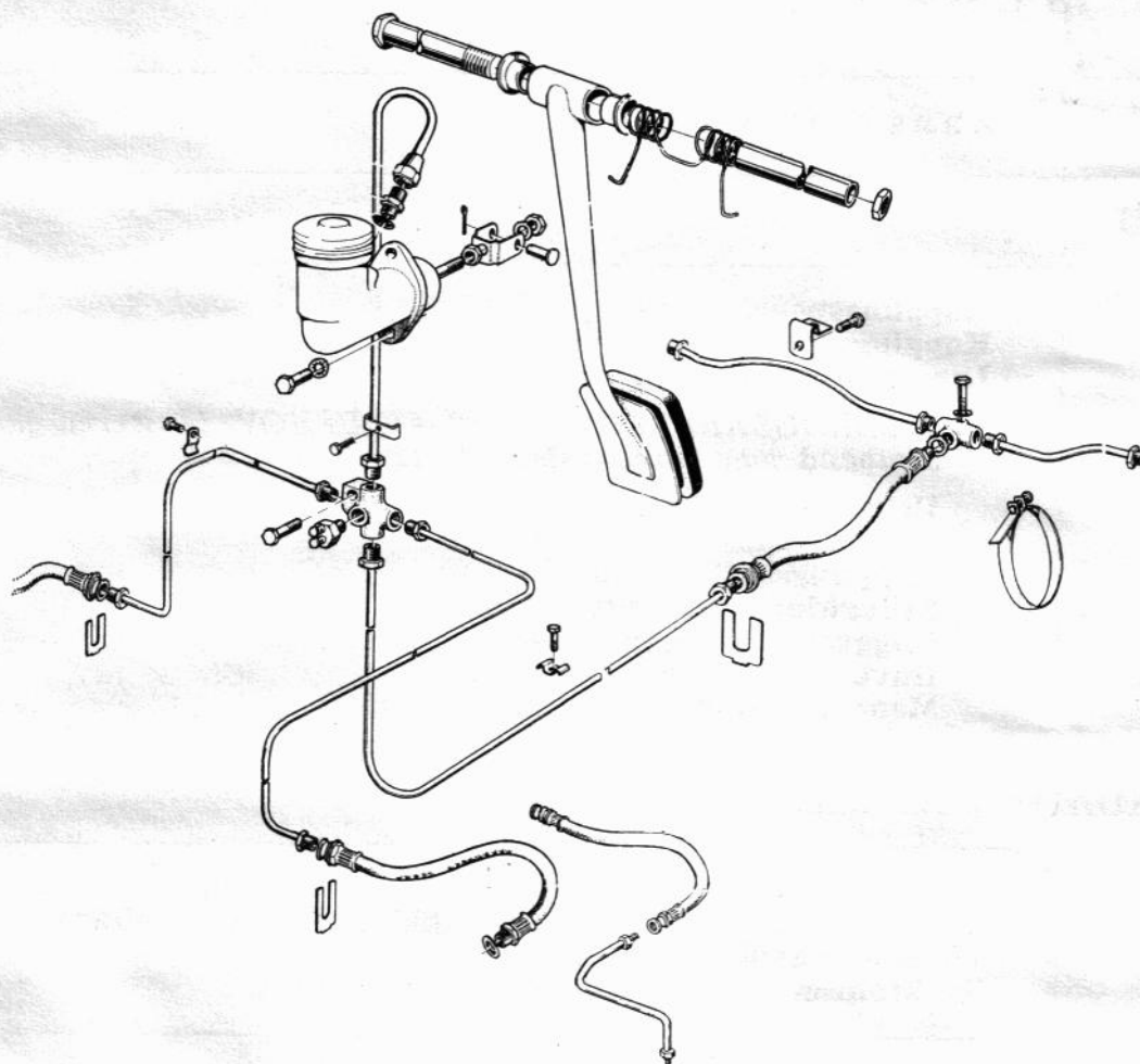
Fotbromsmanövrering
