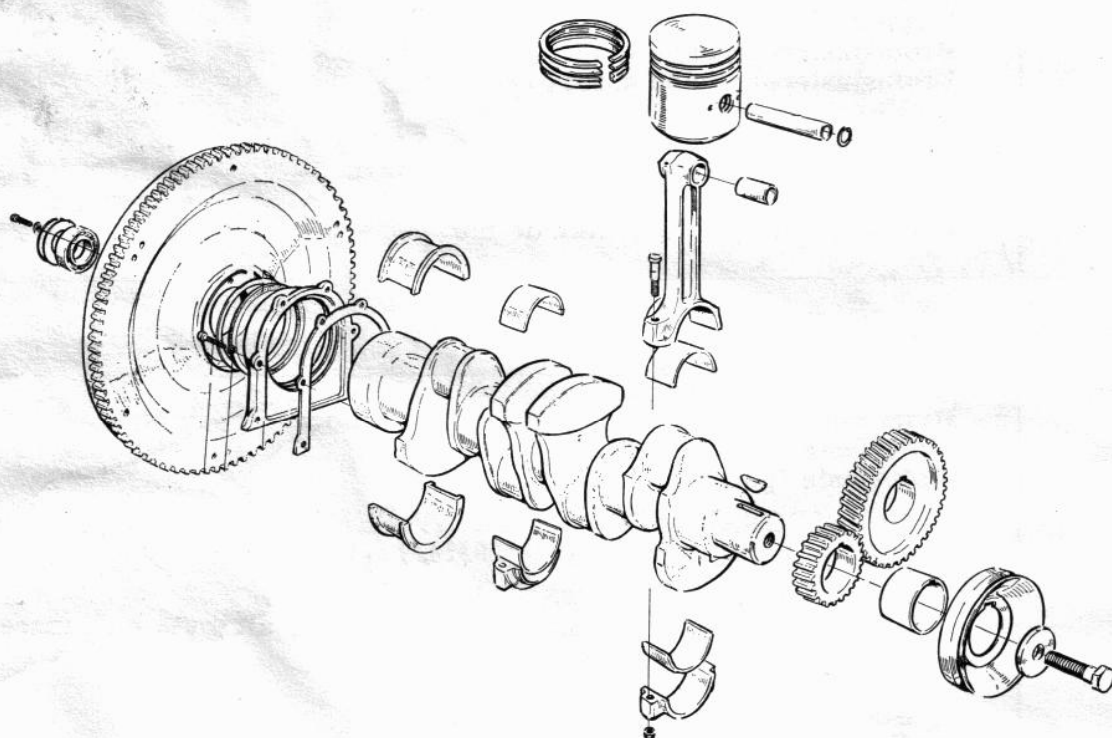
Vevrörelse
