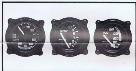
INSTRUMENT "JET-COCKPIT"-SERIEN Varvraknare, oljetryckmätare, oljetemperaturmätare, voltmätare och yttre temperaturmätare. (T.o.m. 1972 års modell.) Se även högra bilden.
