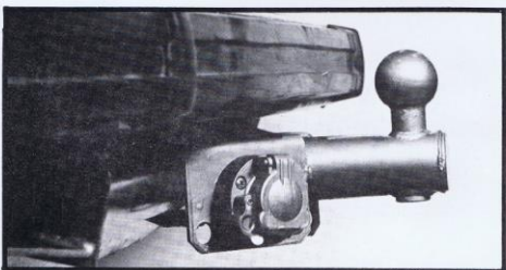
DRAGANORDNING Konstruerad och testad av Volvo.
